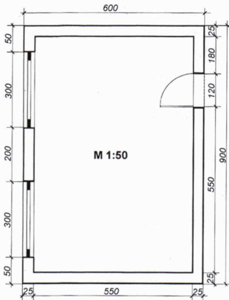
Tehnički crtež tlocrta učionice
